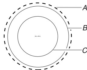
A. Dépassement maximal de \frac{1}{2} " (1,3 cm) B. Bord extérieur de la table de cuisson C. Taille minimale du plat (le cas échéant)
